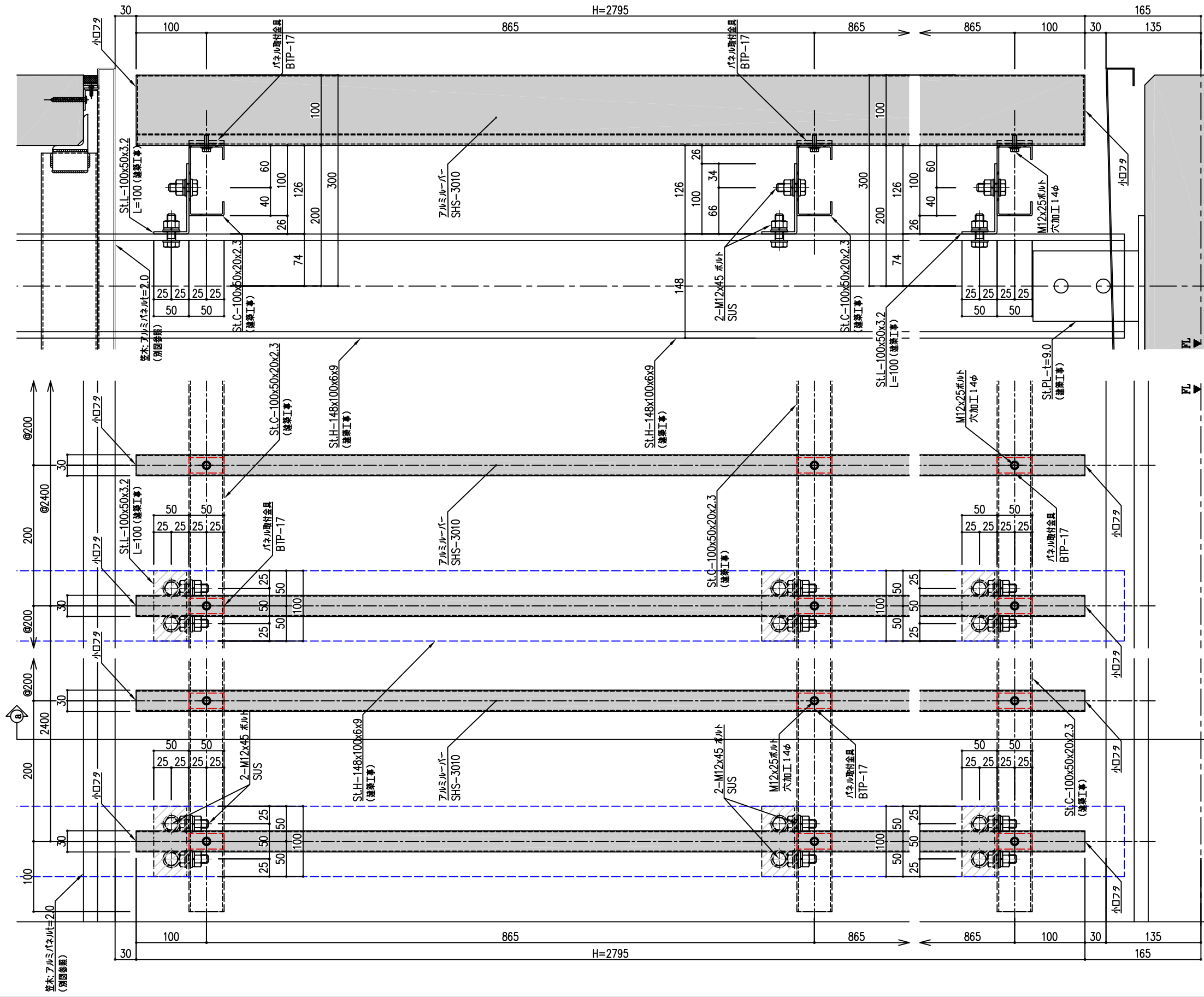
詳細図 A1:1/3 A3:1/6
