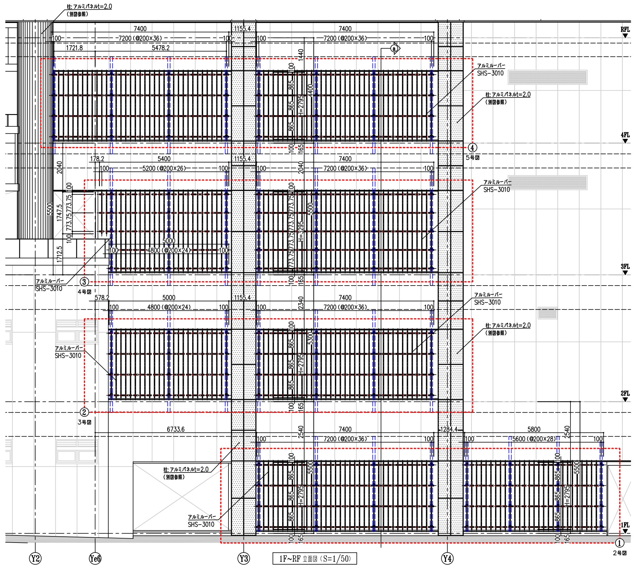
1F~RF 立面図・断面図 A1:1/50 A3:1/100
